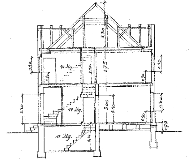
Schnitt a-b
