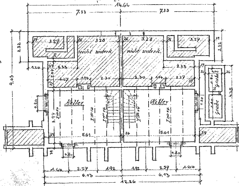
Kellergeschoss
