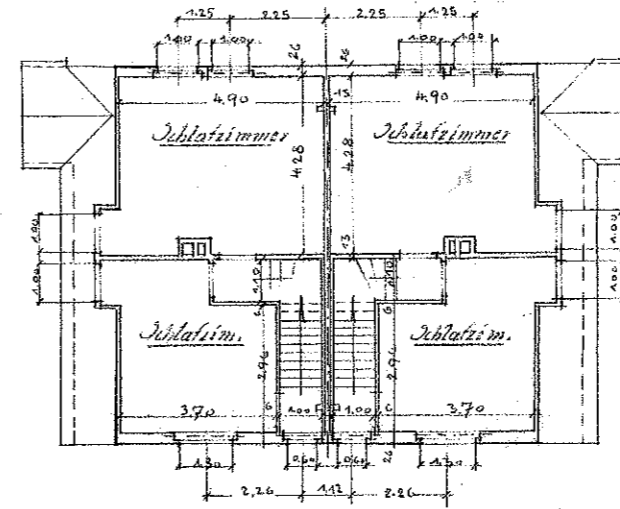
Dachgeschoss
