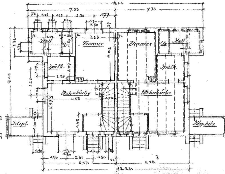
Erdgeschoss
